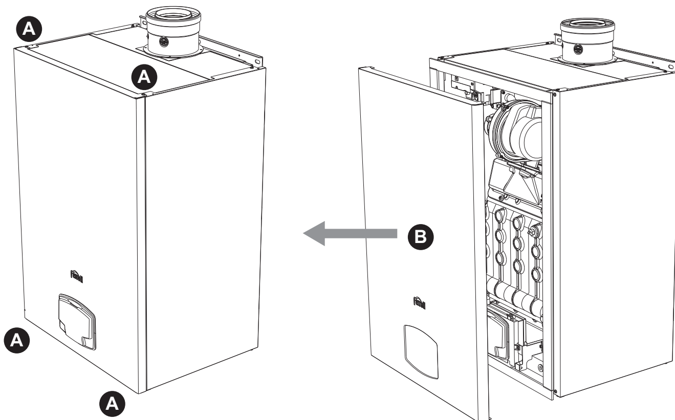
рис. 76- Открытие передней панели
