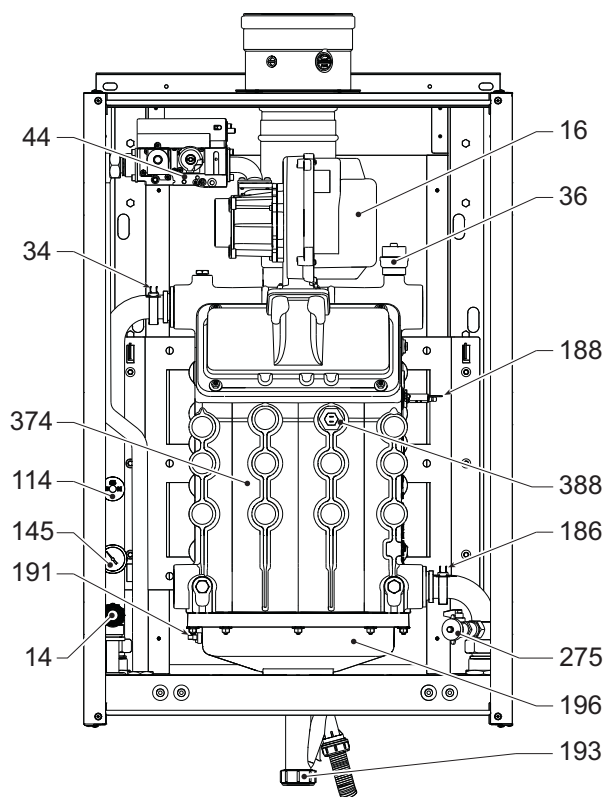
рис. 82- Общий вид, мод. TORO W 99 и TORO W 120
