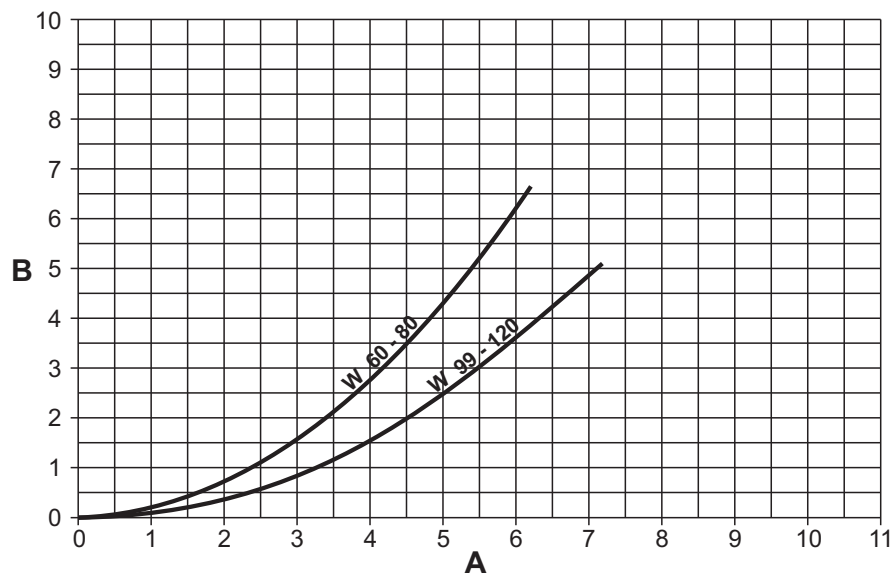
fig. 85 - Diagramma perdita di carico modelli TORO W 60 - TORO W 80 - TORO W 99 - TORO W 120
