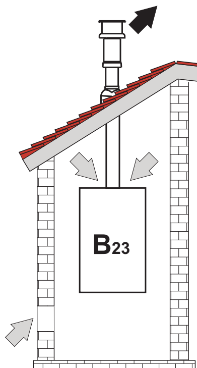
fig. 58- Exemples de raccordement (⇐ = Air / ➡ = Fumées)
