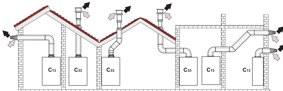
fig. 59- Ejemplos de conexión con tubos coaxiales (⇨ = aire / ⇨ = humos)
