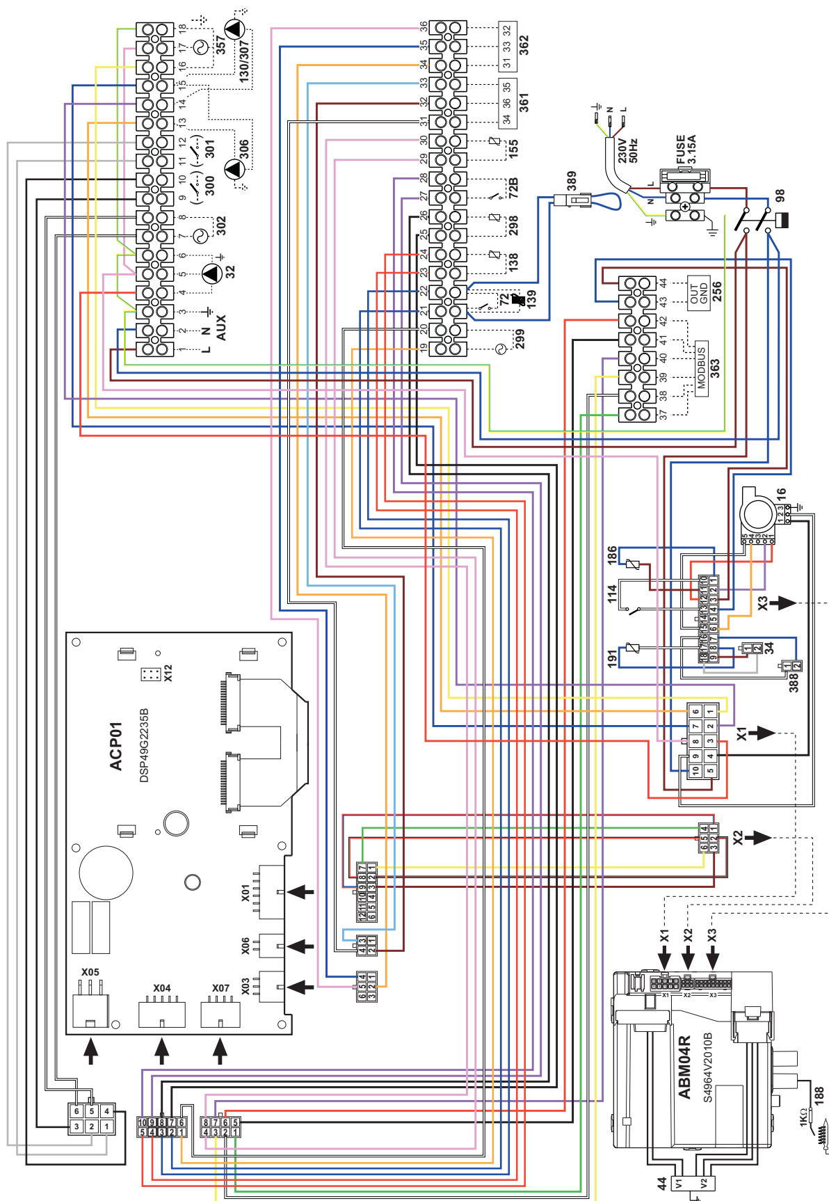
рис. 92- Электрическая схема моделей TORO W 99, TORO W 120 и TORO W 150
