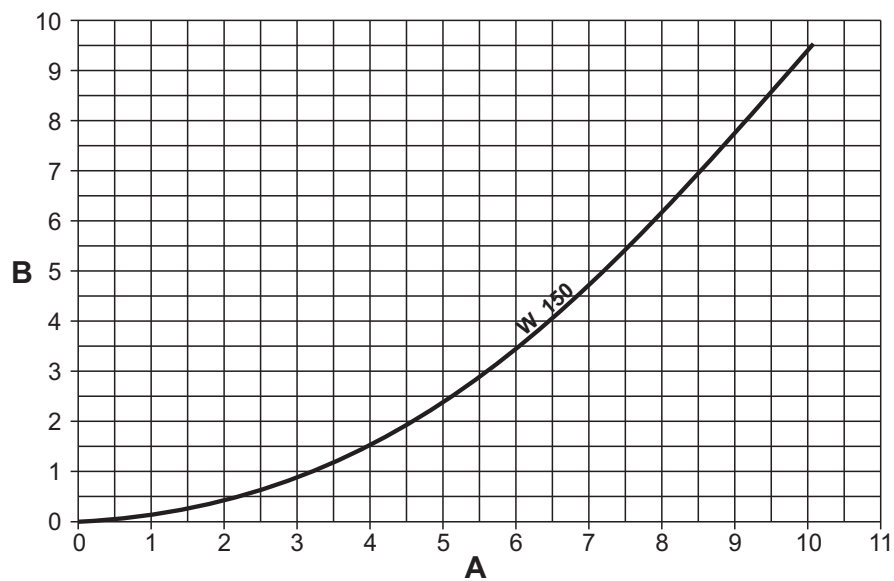
fig. 86 - Diagramma perdita di carico modelli TORO W 150
