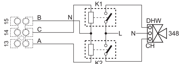
рис. 89- Подключение 3-х ходового клапана с 3 проводами
