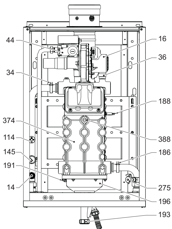
fig. 81- Vista general mods. TORO W 60 y TORO W 80
