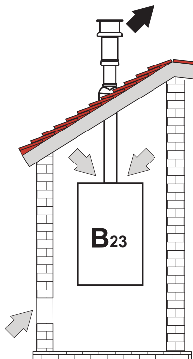
рис. 58- Примеры подключения (⇐= Воздух/ ➡= Дымовые газы)
