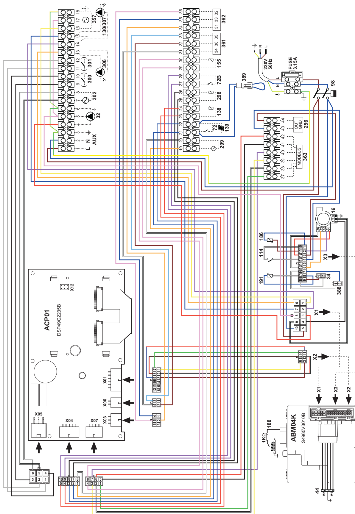
рис. 91- Электрическая схема моделей TORO W 60 и TORO W 80
