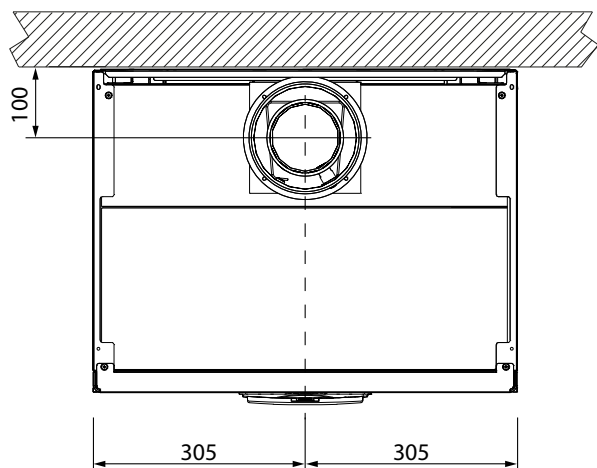
рис. 79- Вид сверху
