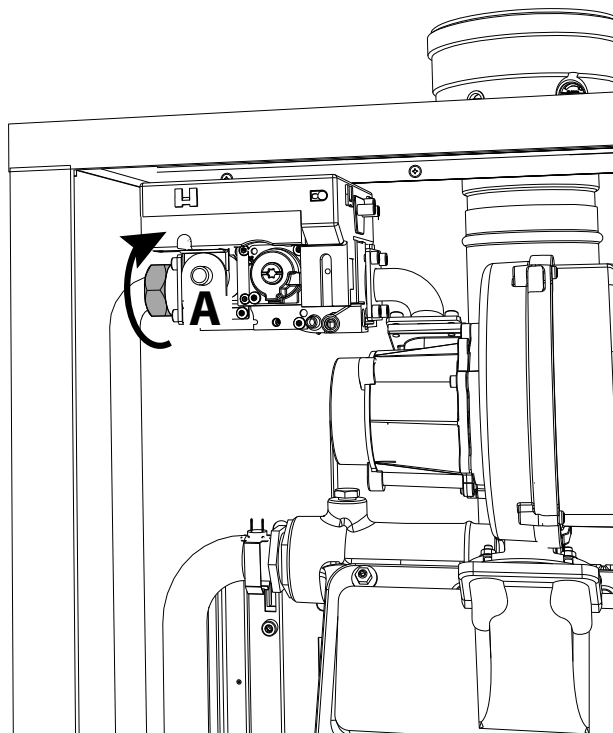
fig. 62- Modèles W 99, W 120 et W 150
