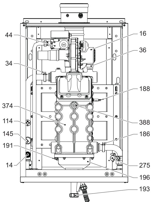
рис. 81- Общий вид, мод. TORO W 60 и TORO W 80
