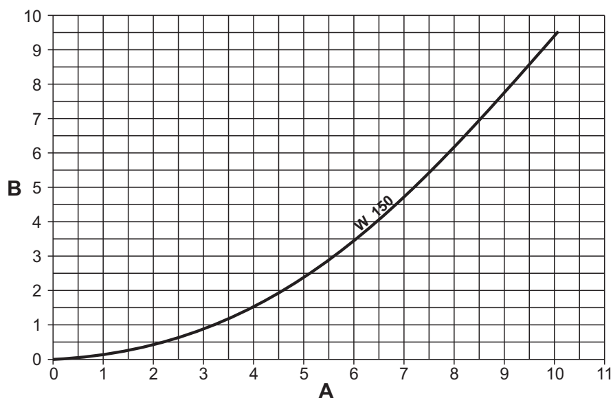
fig. 86- Diagramme perte de charge modèles TORO W 150
