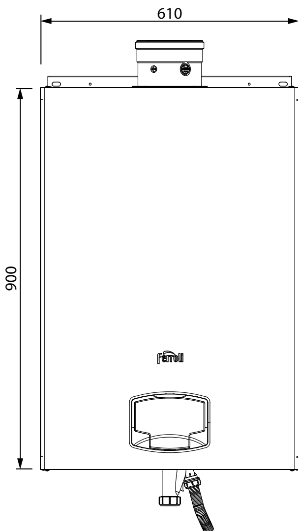
fig. 77- Vue de face
