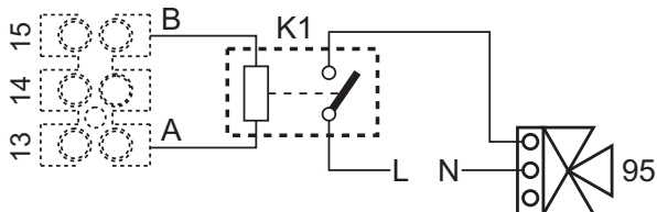
рис. 88- Подключение 3-х ходового клапана с 2 проводами
