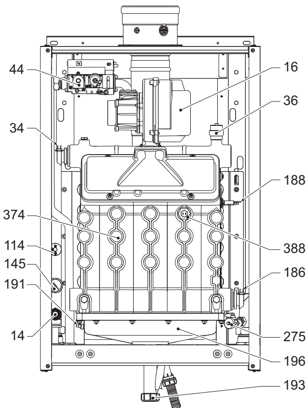
рис. 83- Общий вид, мод. TORO W 150
