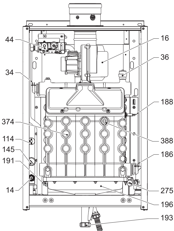
fig. 83 - Vista generale mod. TORO W 150
