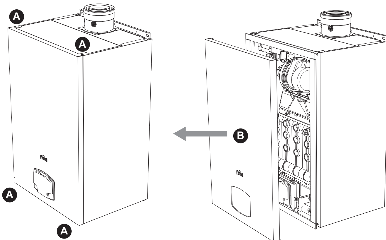
fig. 76- Apertura del panel frontal
