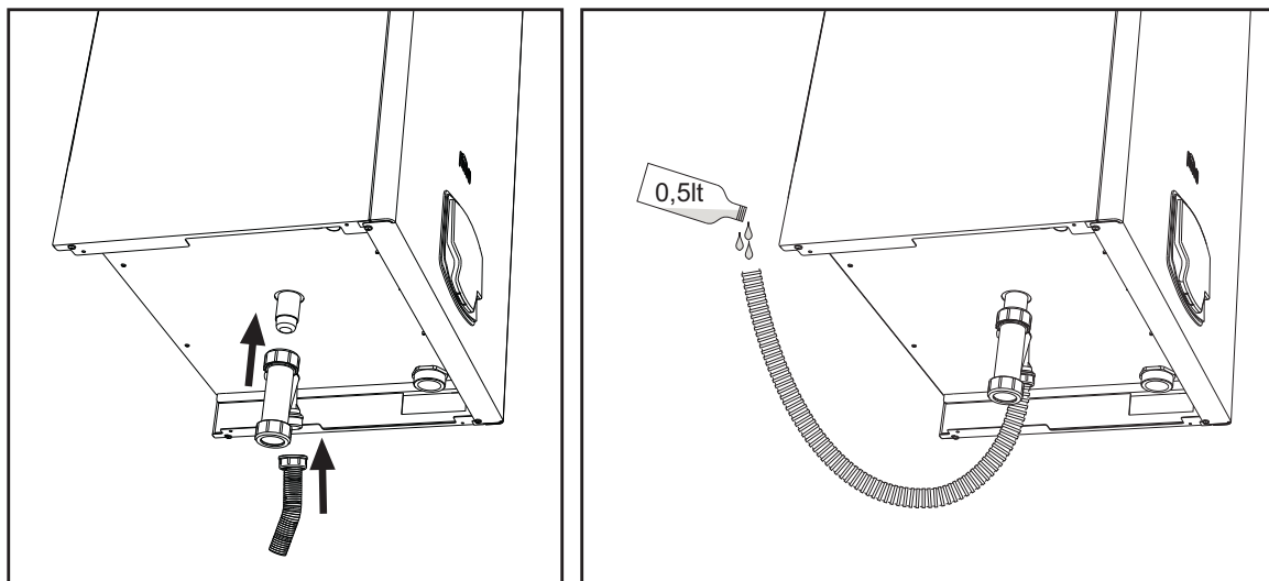
fig. 60 - Collegamento scarico condensa
