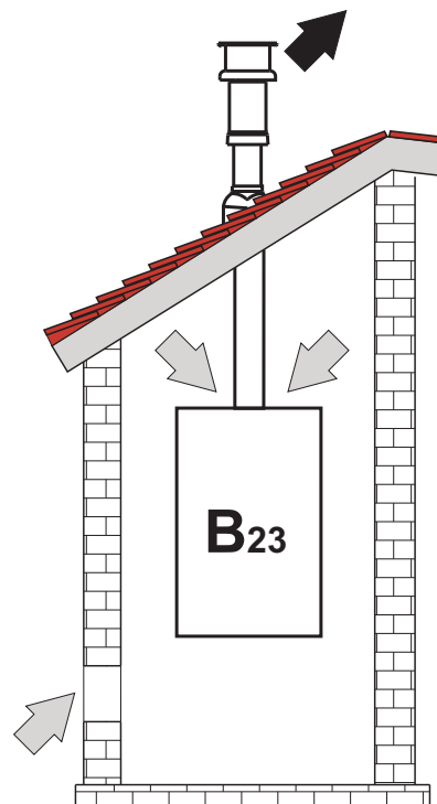
fig. 58 - Esempi di collegamento (⇐=Aria / ➡=Fumi)
