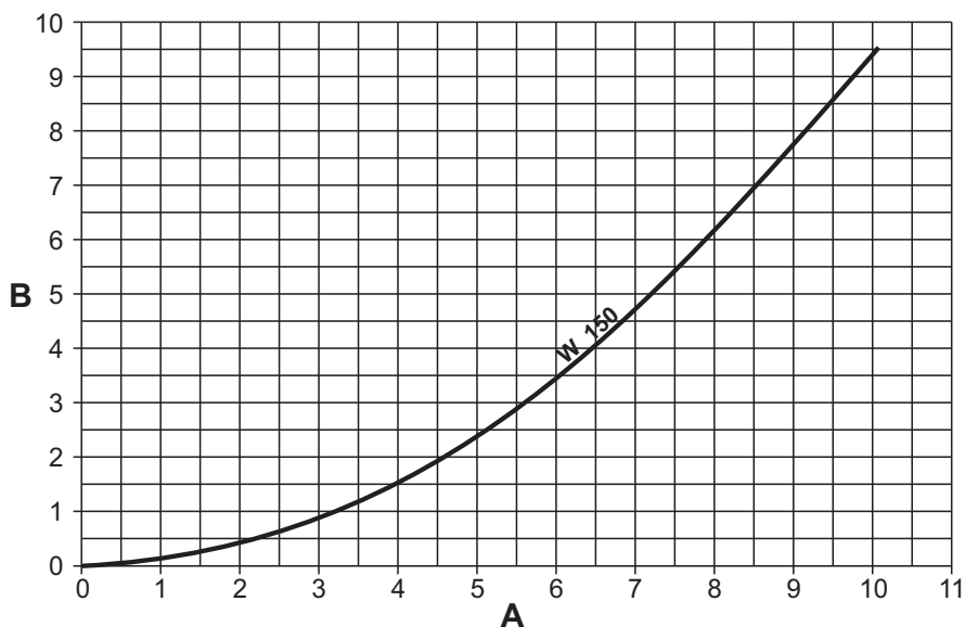
рис. 86- Диаграмма потери нагрузки для моделей TORO W 150
