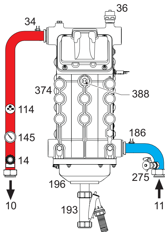
fig. 84- Circuit hydraulique
