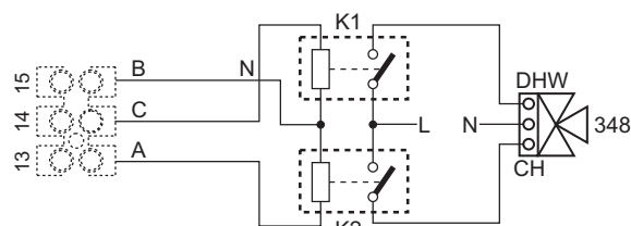
fig. 89- Raccordement de la vanne 3 voies à 3 fils
