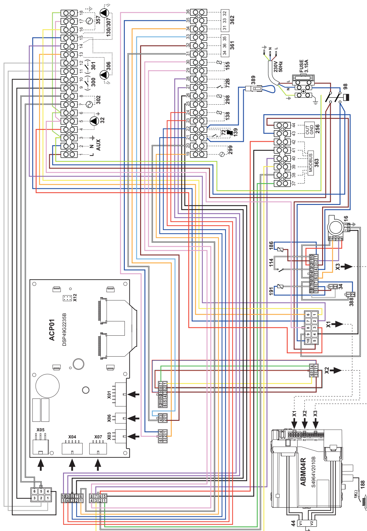
fig. 92 - Schema elettrico modelli TORO W 99, TORO W 120 e TORO W 150
