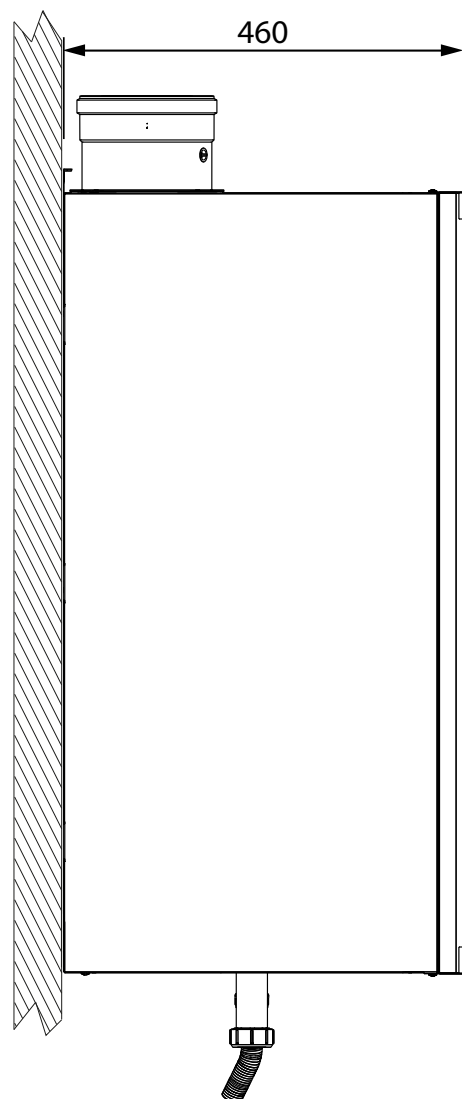
fig. 78- Vue latérale
